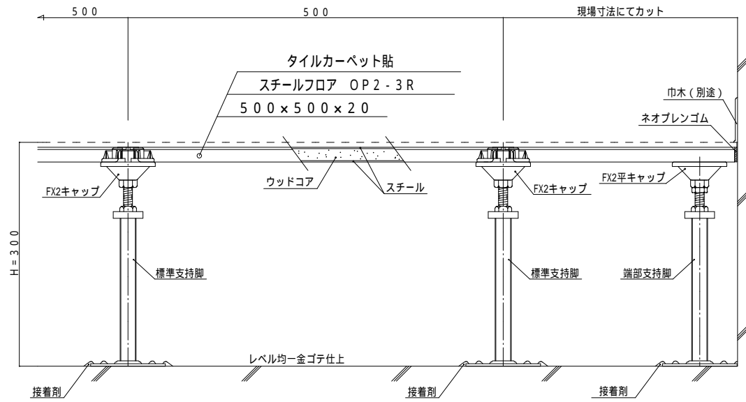
断面図 S = 1 : 5
