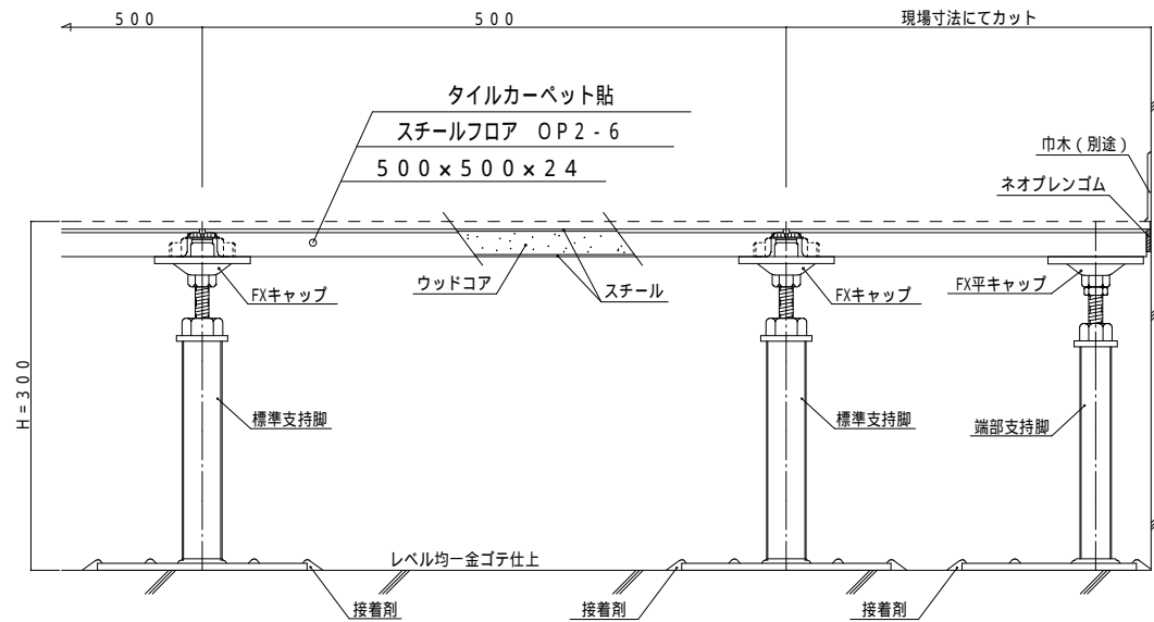
断面図 S = 1 : 5
