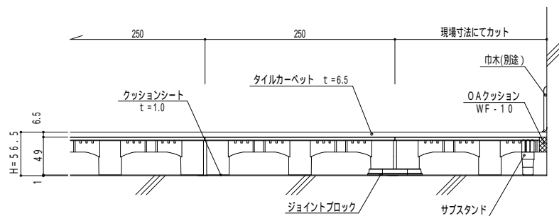
断面図 S = 1 : 5
